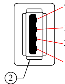
USB A/F
